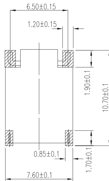
P.C.B. PATTERN DIMENSION (REF)
