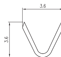
A-A SECTION
