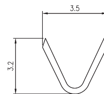
A-A SECTION
